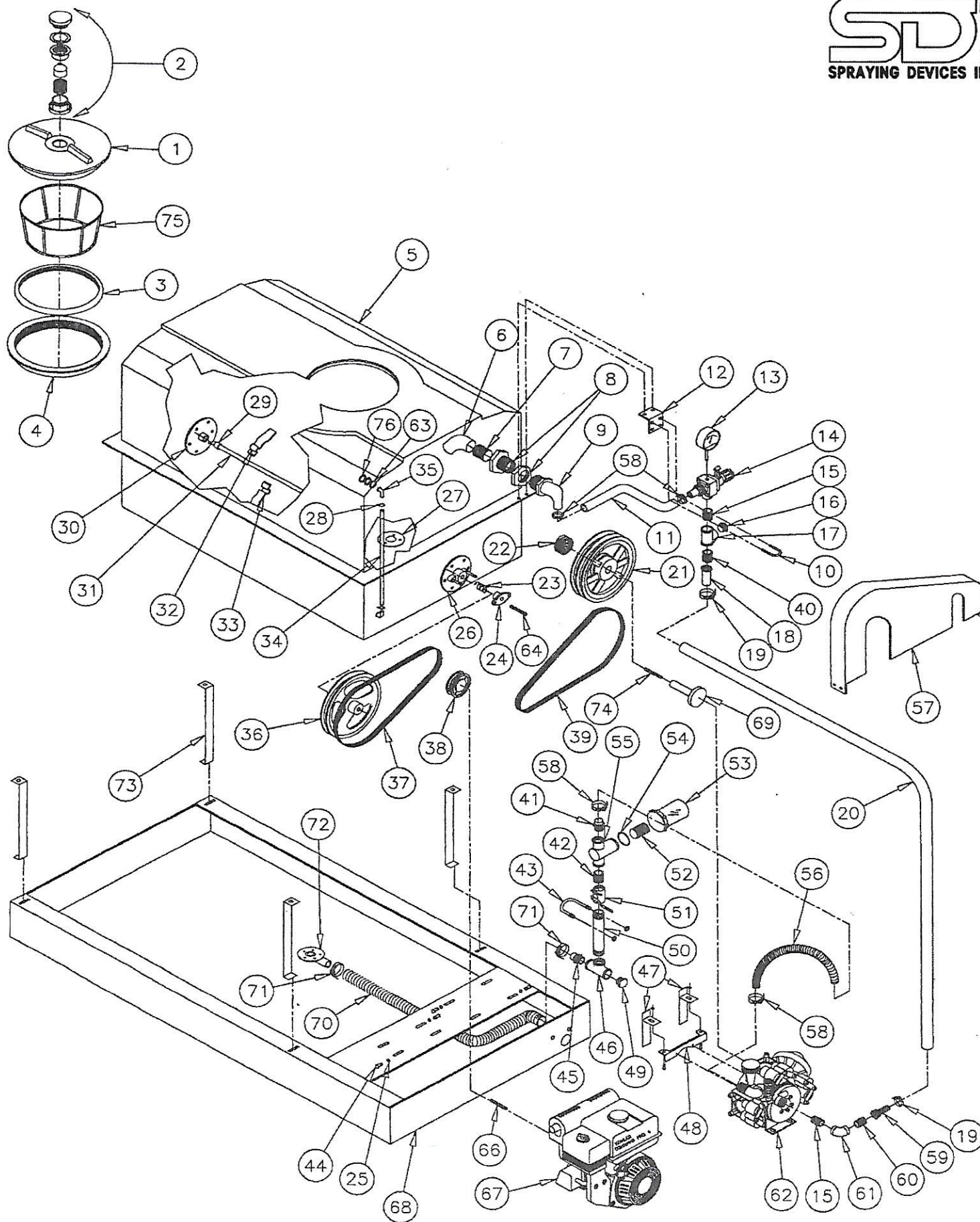
SDI Sprayer-Models TM100/ TM200 and TM300
